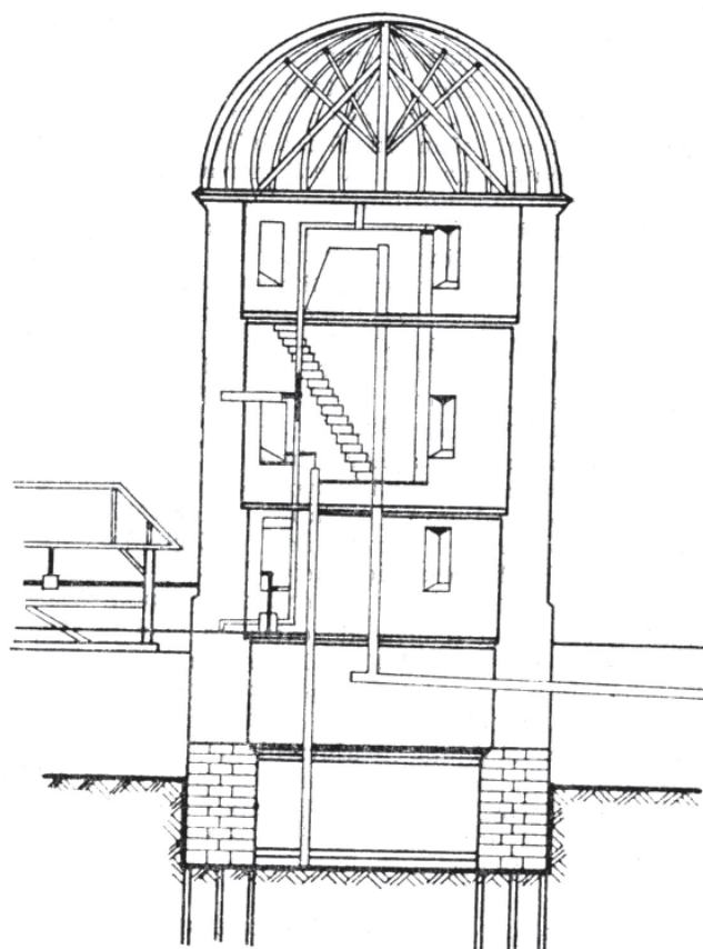
Reconstituire a instalației mecanice de pompare din 1774
